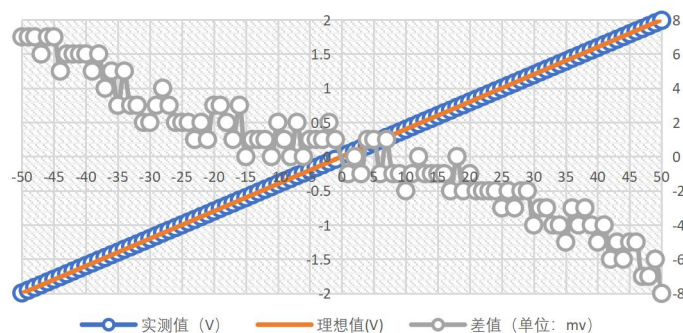
图 5: 输出电压非线性差值
