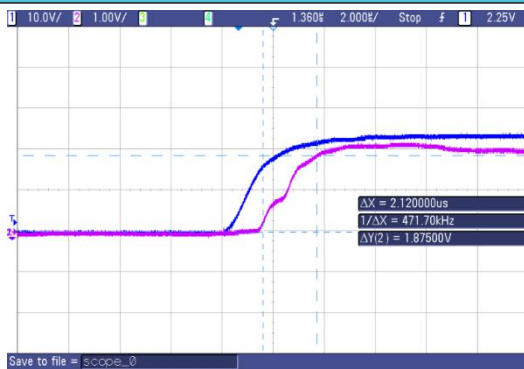
图 3: 响应延迟时间图
